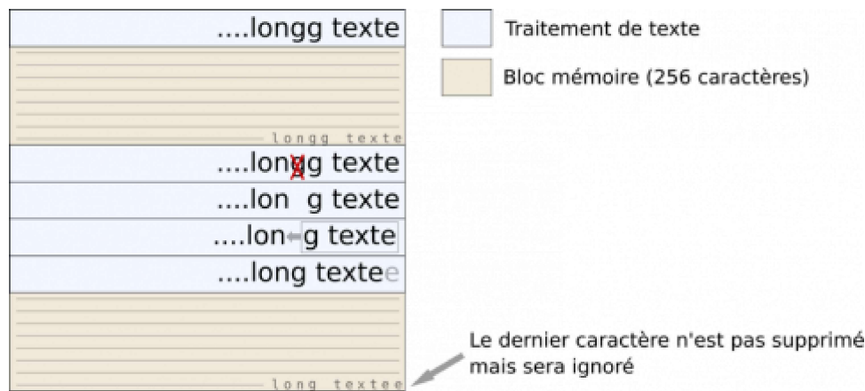
Fig. 4 : Incidence d'une suppression dans le traitement de texte sur un bloc mémoire
